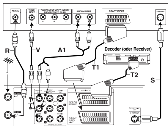
Rückseite dieses Geräts (Grundanschluss)
