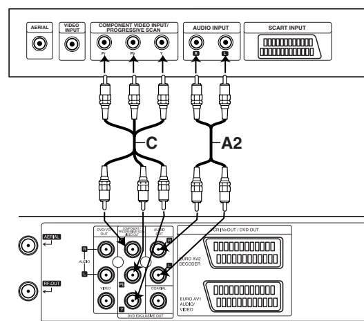
Rückseite dieses Geräts (Anschluß des DVD-Ausgangs)
