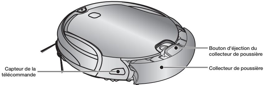
Face latérale
