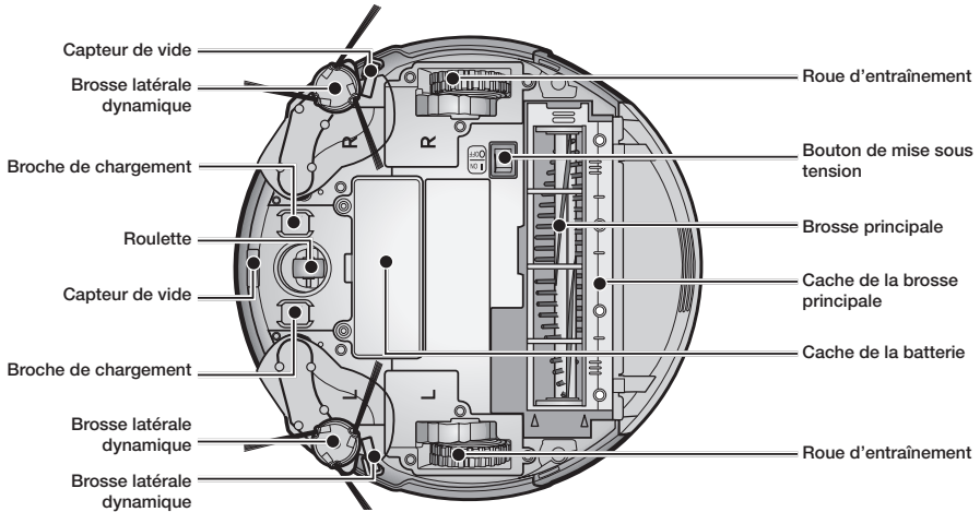
Dessous
