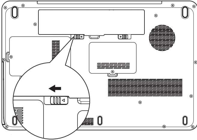
Abbildung 6-1 Akku entsichern (1)
