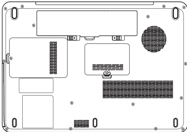
Abbildung 8-3 Speichermodulabdeckung einsetzen
