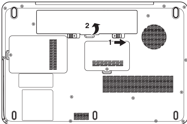
Abbildung 6-2 Akku entsichern (2)
