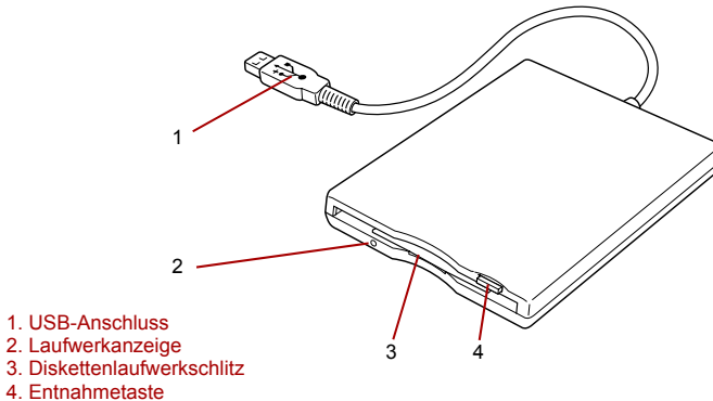
Abbildung 8-4 USB-Diskettenlaufwerk
