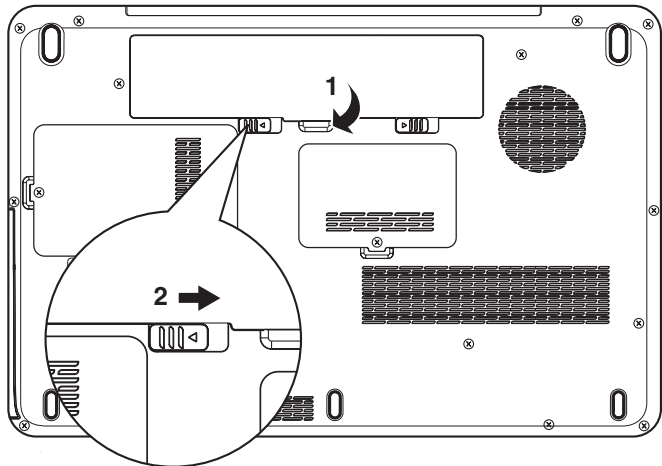
Abbildung 6-3 Sichern des Akkus
