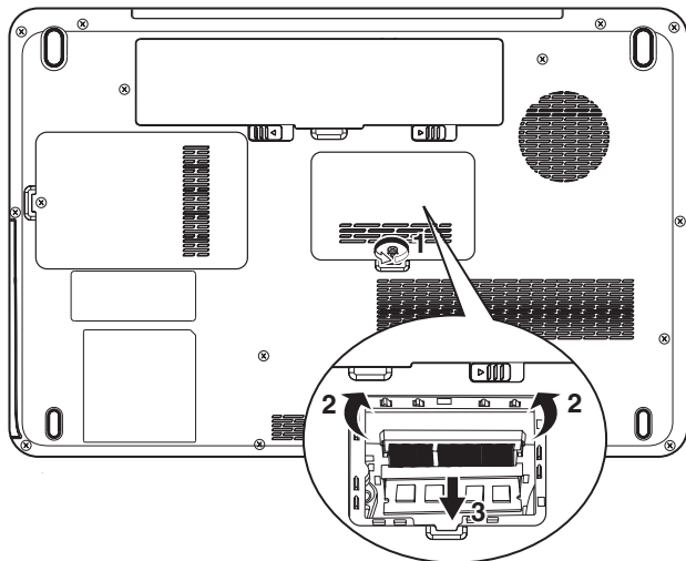
Abbildung 8-2 Speichermodul-Abdeckung entfernen
