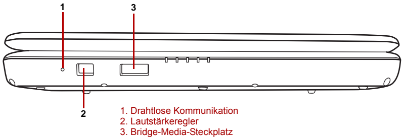
Abbildung 2-1 Vorderseite des Computers mit geschlossenem Bildschirm
