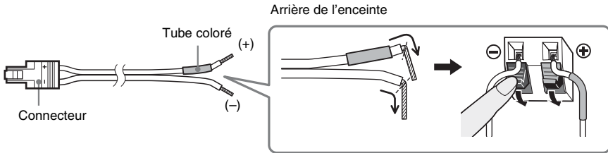
Panneau arrière
