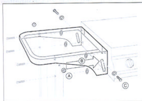
Montage des Seitentablers
