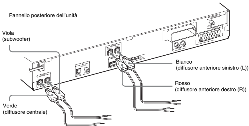
Pannello posteriore dell'amplificatore surround
