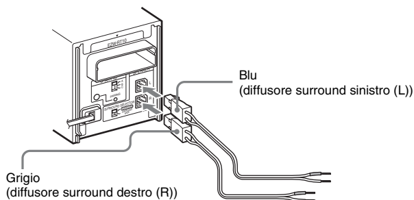
Pannello posteriore dell'amplificatore surround
