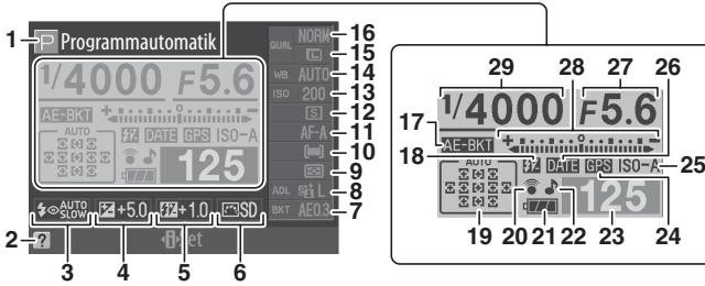
Kamera in normaler Bildausrichtung
