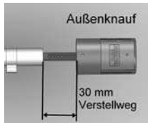
Schematische Darstellung Außenknauf-Verstellung
