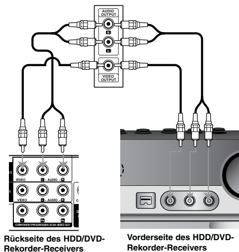
Anschlussleiste für Zusatzgeräte (Videorekorder, Camcorder usw.)
