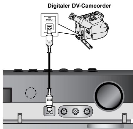
Vorderseite des HDD/DVD-Rekorder-Receivers
