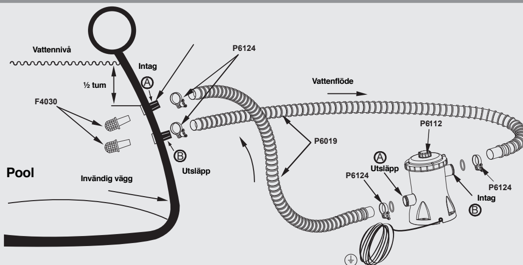
Illustration (inte i skala) av poolen och filterpumpen ROUCHER™
