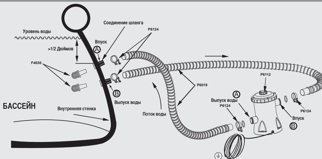
Иллюстрация(без соблюдения масштаба) бассейна и фильтрационного насоса КОЛЕСИКАР™
