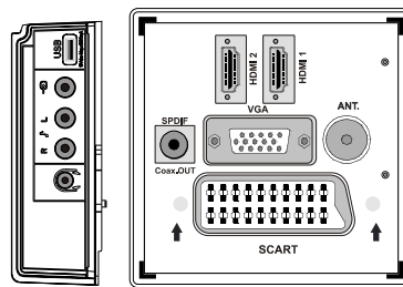
Audioeingänge des TV-Geräts
