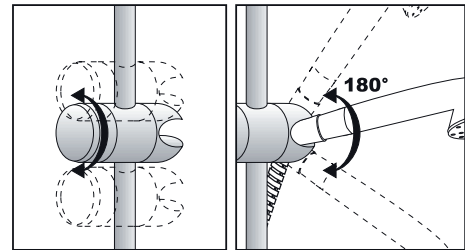
CURSEUR POUR BARRE MURALE CURSOR PARA BARRA MURAL CURSOR PARA BARRA DE PAREDE
