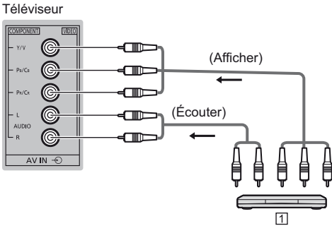
1 Lecteur DVD
