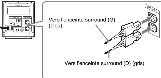
Panneau arrière de l'amplificateur surround
