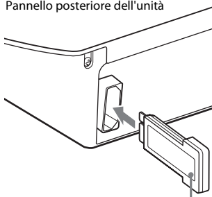
Transricevitore wireless
