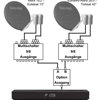
Beispiel 3: 4 Satelliten (Quattro-LNBs) Astra 19,2°/ Eutelsat 13° Eurobird-Astra 28,5°/ Türksat 42°
