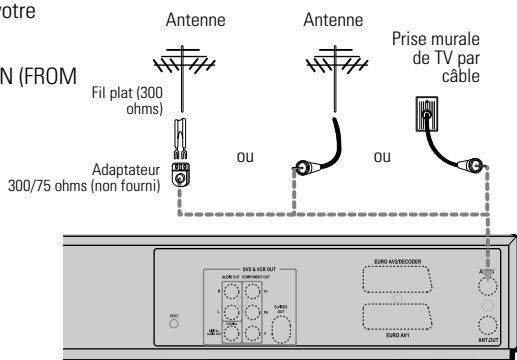
Arrière du combiné Graveur DVD + Magnéscope
