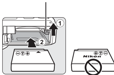
Blocco batteria
