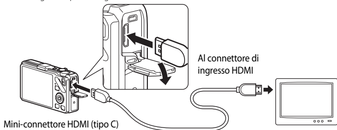
Mini-connettore HDMI (tipo C)
