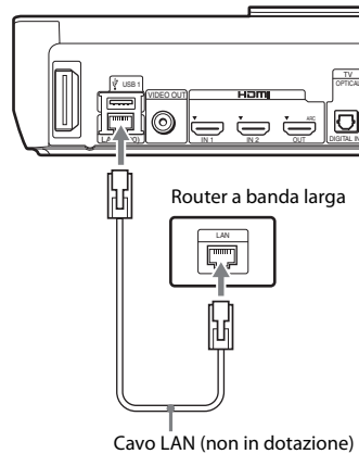
Pannello posteriore dell'unità
