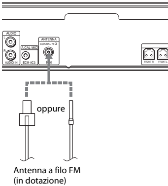
Pannello posteriore dell'unità
