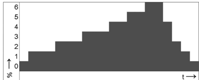
P1: Hellingshoekprofiel 2
