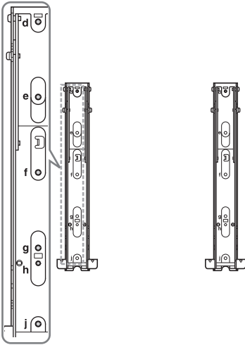
Emplacement des vis
