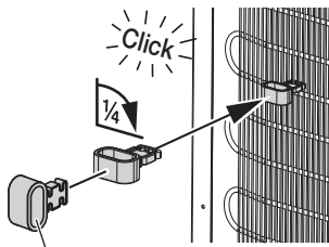
Wandabstandshalter
