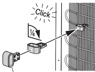
distanciateur
