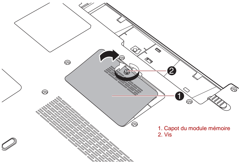
Illustration 3-8 Retrait du capot du module mémoire
