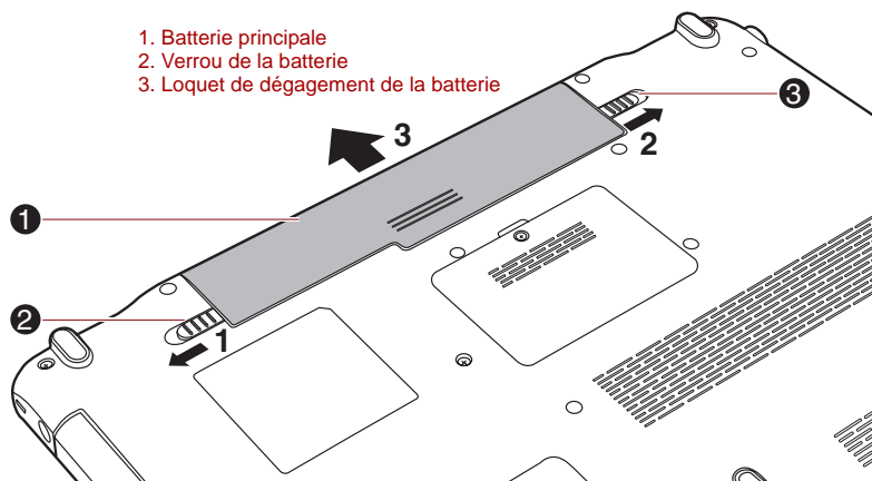
Illustration 6-1 Retrait de la batterie
