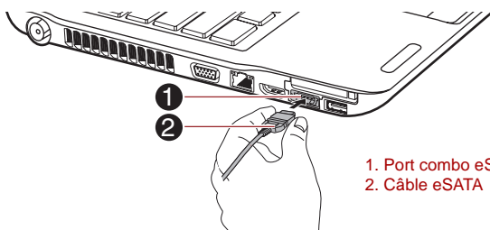
Illustration 3-13 Connexion d'un câble eSATA sur le port mixte eSATA/USB
