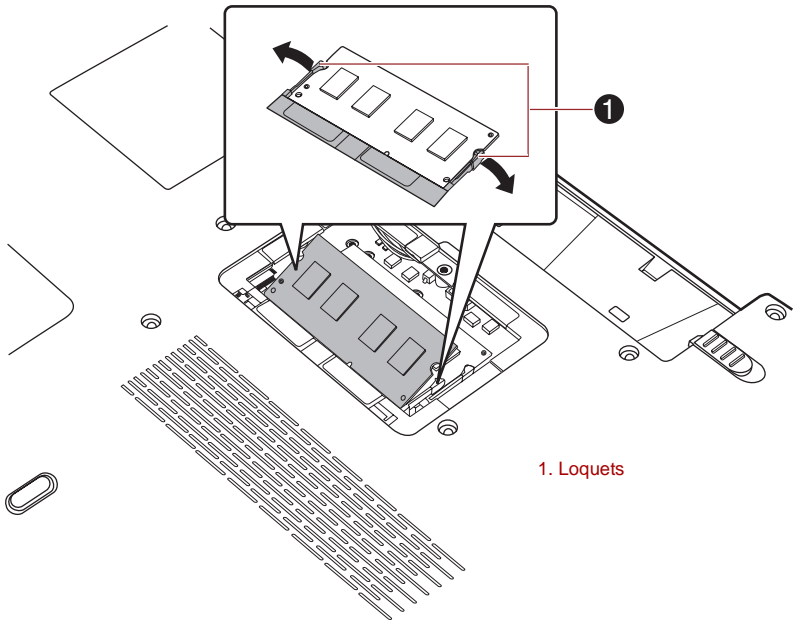
Illustration 3-9 Retrait d'un module mémoire
