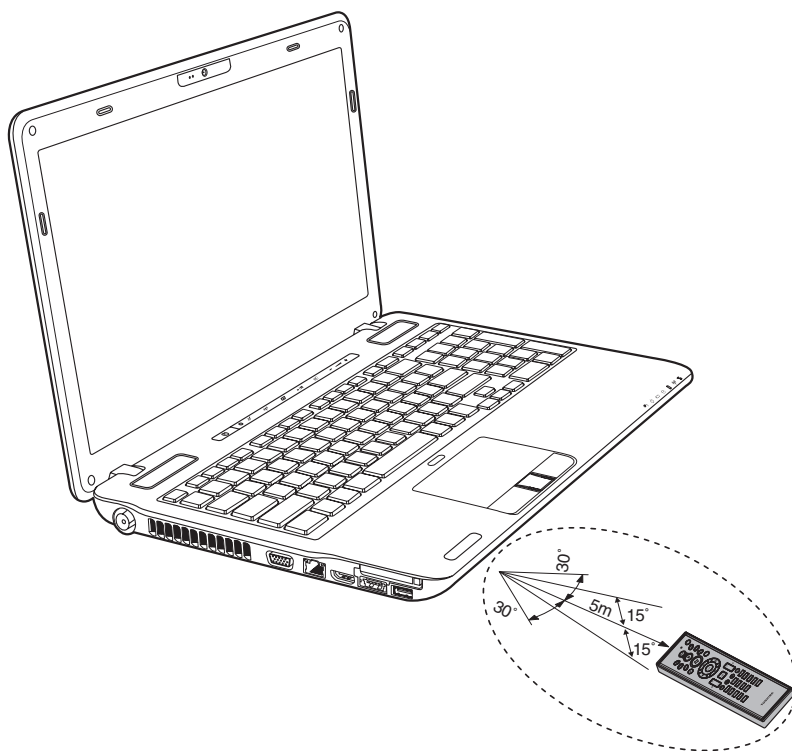
Illustration 2-12 Zone de portée de la télécommande
