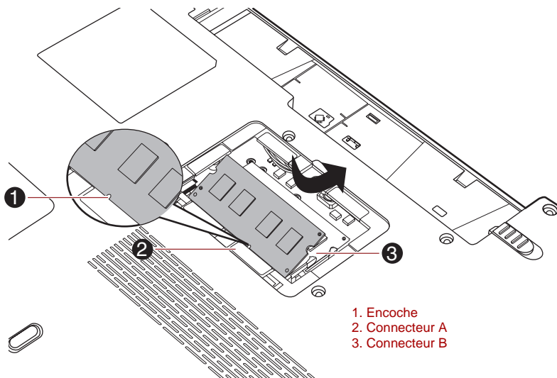
Illustration 3-7 Pose du module mémoire
