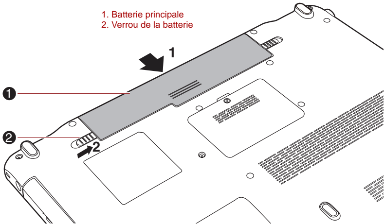
Illustration 6-2 Verrouillage de la batterie
