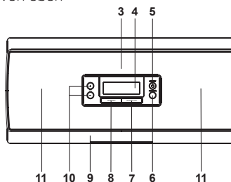
Vorderansicht
