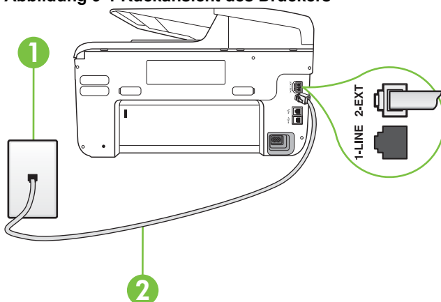
Abbildung 9-1 Rückansicht des Druckers
