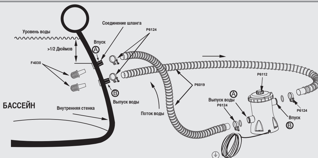
Иллюстрация(без соблюдения масштаба) бассейна и фильтрационного насоса POLESTAR™
