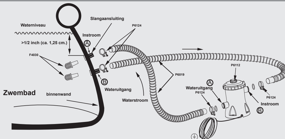
Tekening (niet op schaal) van zwembad en ROUCLAR™ filterpomp
