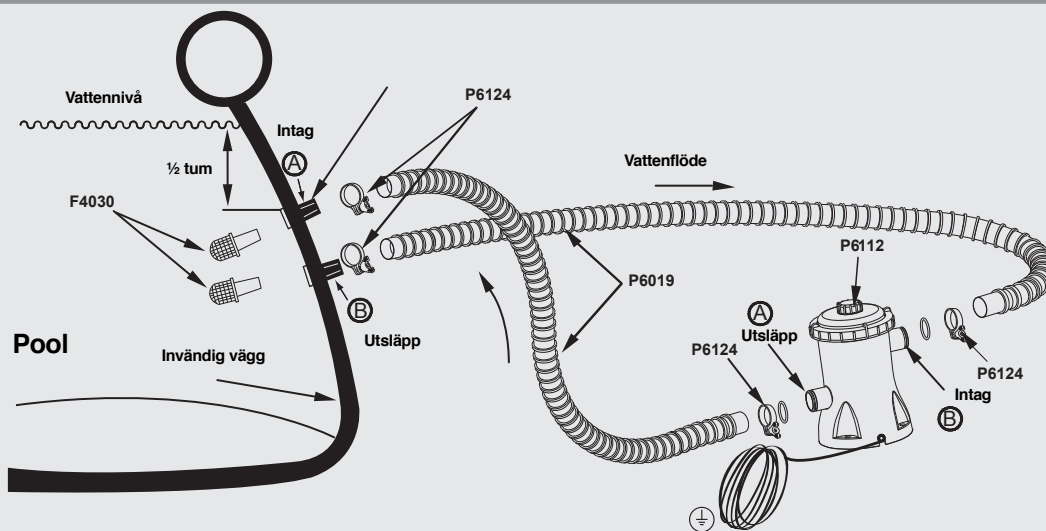
Illustration (inte i skala) av poolen och filterpumpen POOLCARE™
