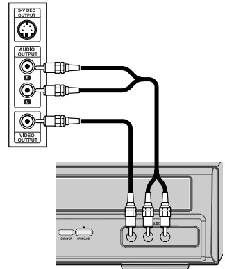
Avant du combiné Graveur DVD + Magnéscope
