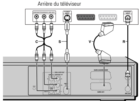
Arrière du combiné Graveur DVD + Magnéscope
