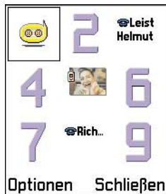
Abb. 3 Die Kurzwahlübersicht
