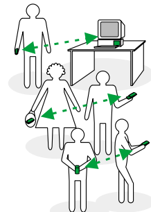
Abb. 1 Bluetooth verwenden.
