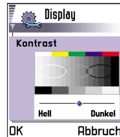
Abb. 1 Ein Einstellungsregler.
