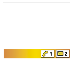
Abb. 3 Der Bildschirmschoner.
