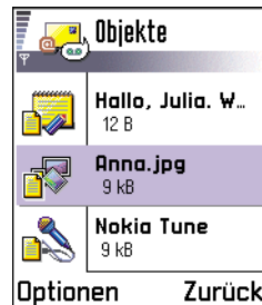
Abb. 5 Multimediaobjektansicht.
