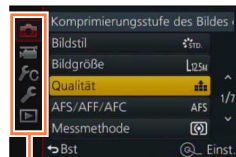
Menütyp
