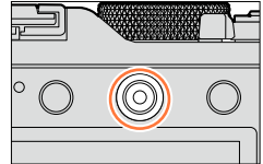
Aufnahmestatus-Anzeige
