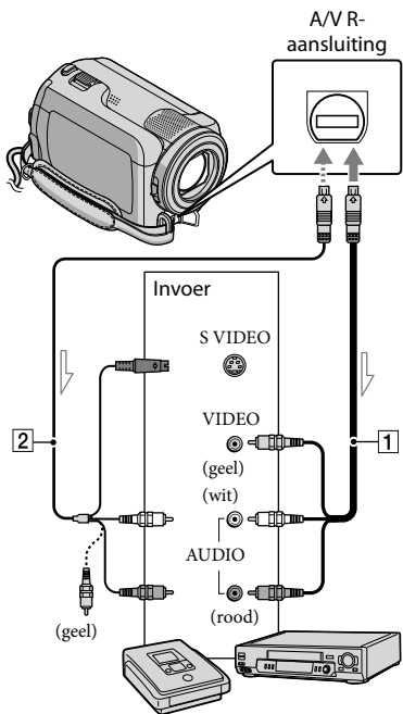
➡ Signaalverloop
