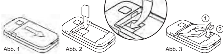
Abb. 1: Akkudeckel entfernen (wie abgebildet). Abb. 2: SIM-Karte mit den goldenen Kontakten nach unten einlegen.
