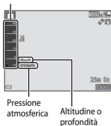
Altimetro o profondimetro
