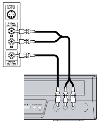
Frontale dell'apparecchio
