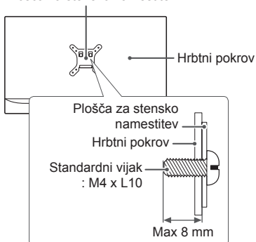
Plošča za stensko namestitev
