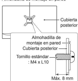
Almohadilla de montaje en pared
