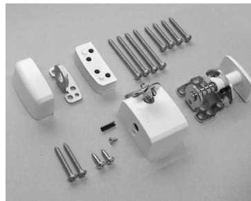
DIN gauche DIN links DIN izquierdo côté serrure Sluitzijde parte del cerrojo
