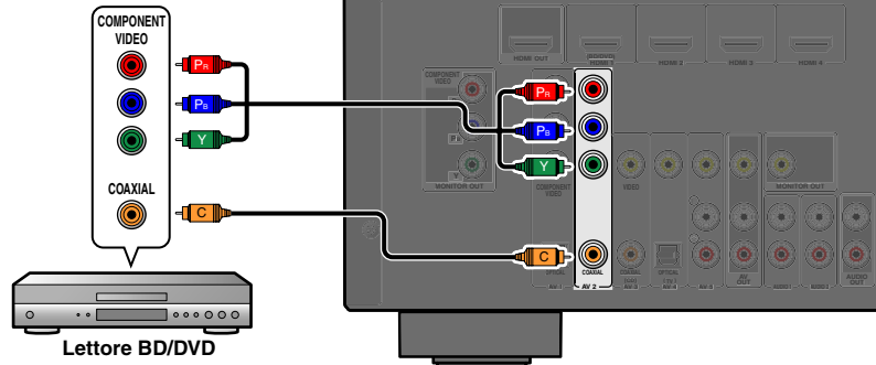
Uscita video a componenti / Audio (coassiale)
