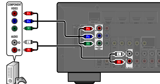
Uscita video a componenti / Audio
