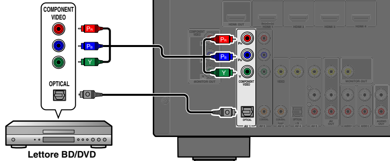
Uscita video a componenti / Audio (ottica)
