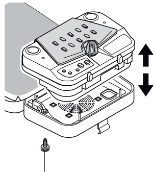
Befestigungsschrauben lösen
