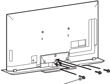
Bevestigingsschroef nek tv-standaard (M5 × 16)
