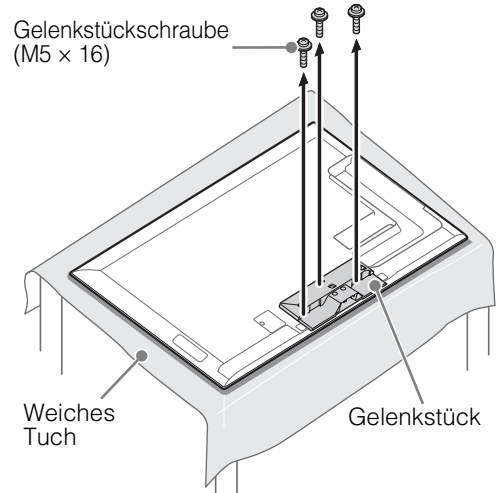
Befestigungsschraube des Ansatzstücks für den Fernsehständer (M5 x 16)
