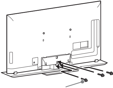
Befestigungsschraube des Ansatzstücks für den Fernsehständer (M5 x 16)
