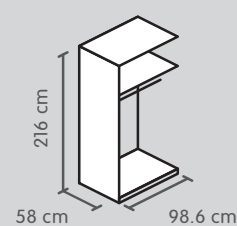
Élément additionnel 100 cm
