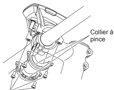
Boulon du collier à pince
