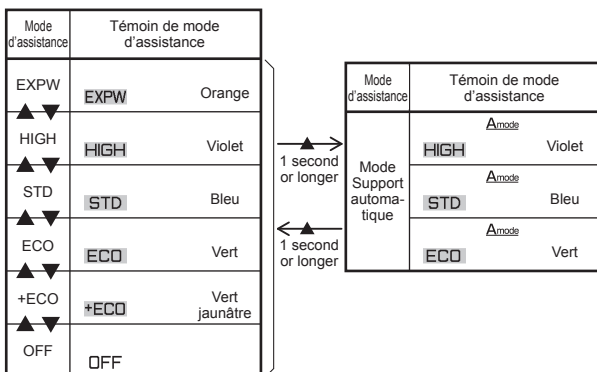
Unité d'entraînement PW-X2
