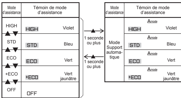
Unité d'entraînement PWseries TE
