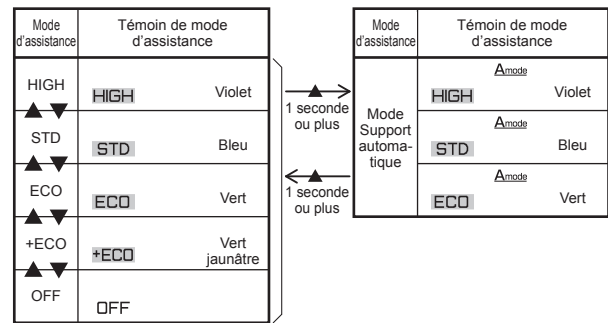
Unité d'entraînement PWseries ST
