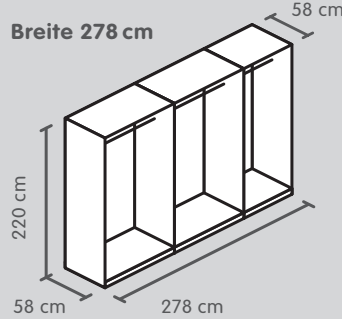
6 Paneele à 75 cm 3 Paneele à 125 cm
