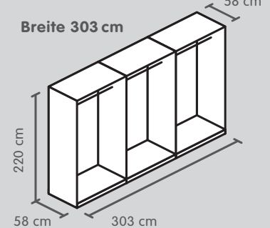
9 Paneele à 100 cm
