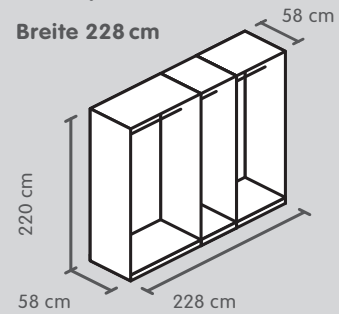
9 Paneele à 75 cm
