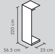
Anbauelement 25 cm 1 Kleiderstange
