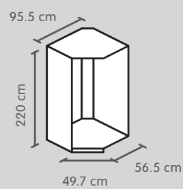
Eckanbauelement 1-türig 1 Kleiderstange
